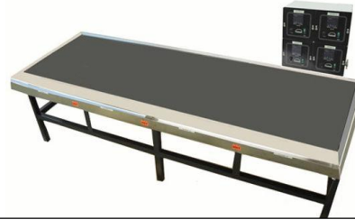
(上图) 均匀粘合台, 36 x 144 英寸, 4 个区域由数字恒温器控制。
